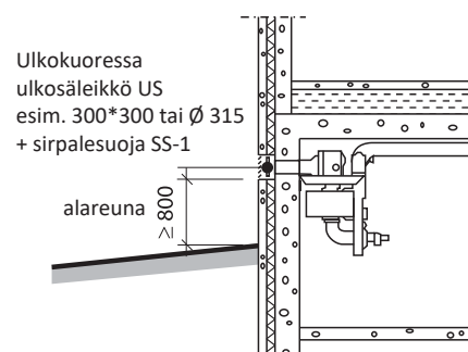
LP-1P IVL -laitteiston läpivienti, korkeus
